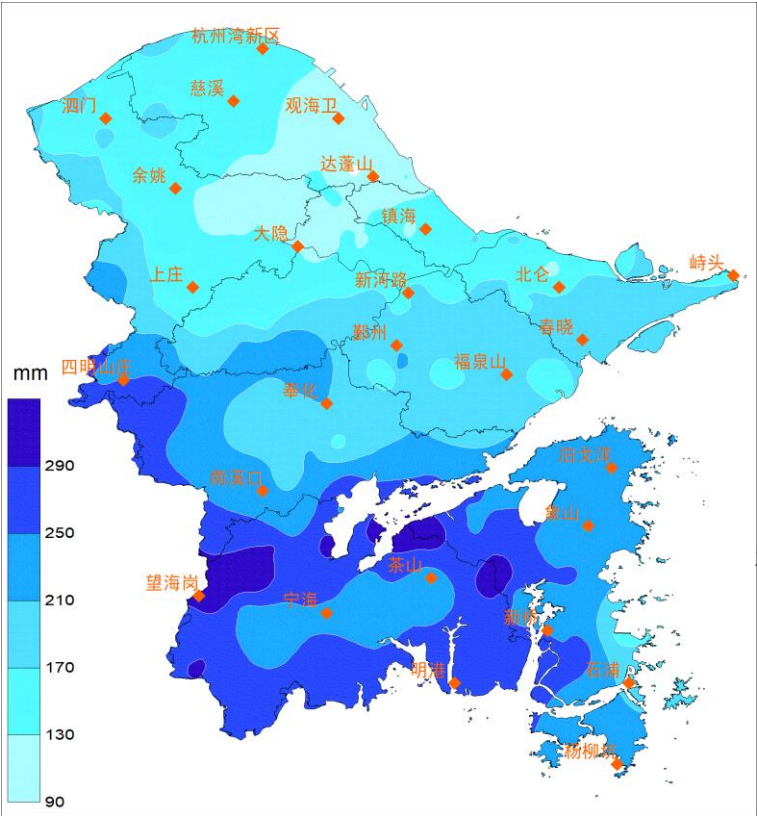
宁波市 2021 年 5 月降水量空间分布图
