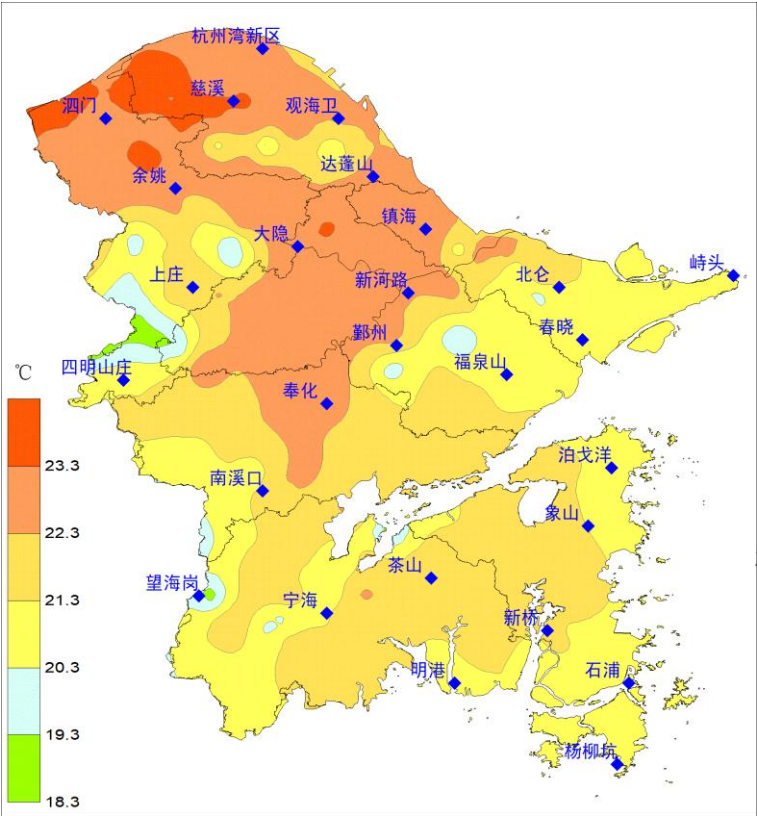
宁波市 2021 年 5 月平均气温空间分布图
