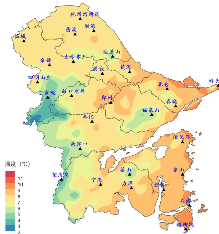
宁波市 2024 年 12 月平均气温空间分布图
