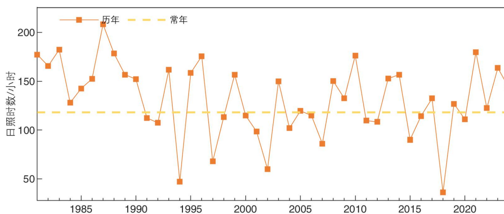
宁波市 12 月日照时数年际变化图
